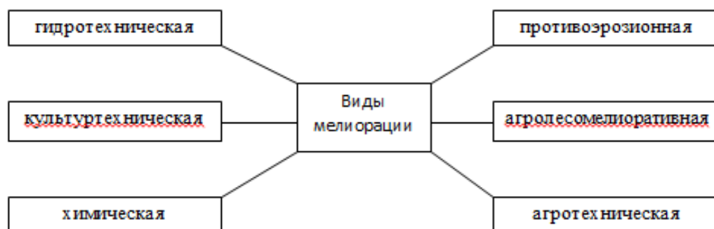
Рис.1 Виды мелиорации
