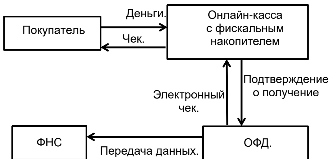
Рис. 1. Принцип работы онлайн-кассы.
